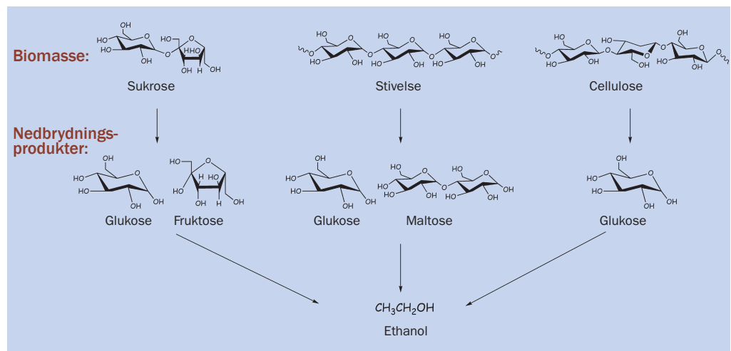
Figur 1. Nedbrydningsprodukter fra forskellige biomasser, der kan omdannes til ethanol.
