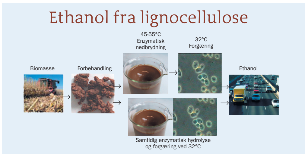
Figur 2. Procesdesign ved separat og simultan enzymatisk hydrolyse og forgæring.
